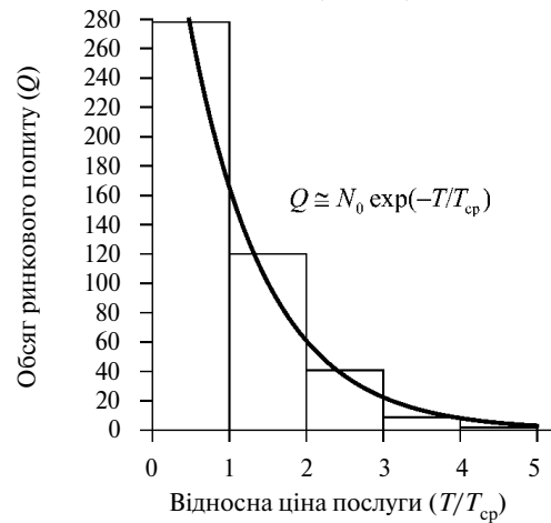
Рис. 2. Емпірична гістограма розподілу незможних людей за розміром бажаних тарифів, віднесених до величини середнього тарифу T_{ср} = 3,8\% (у вигляді стовпців), і асимптотична функціональна залежність обсягу попиту на мікрострахову послугу Q(T) = N_0 \exp(-T/T_{ср}) від ціни страховки P = T/T_{ср} (у вигляді неперервної спадної кривої)
