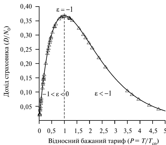
Рис. 4. Дохід страховика залежно від ціни P для нееластичного та еластичного ринкового попиту
